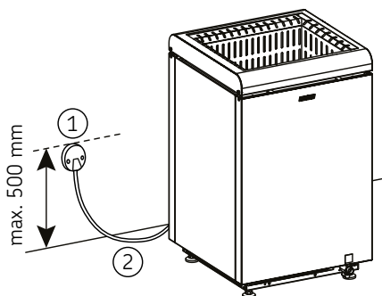
Obrázek 4 Elektrické připojení
