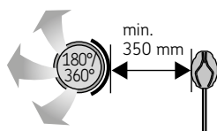
Rysunek 10. Minimalna odległość otworu wentylacyjnego od czujnika.
