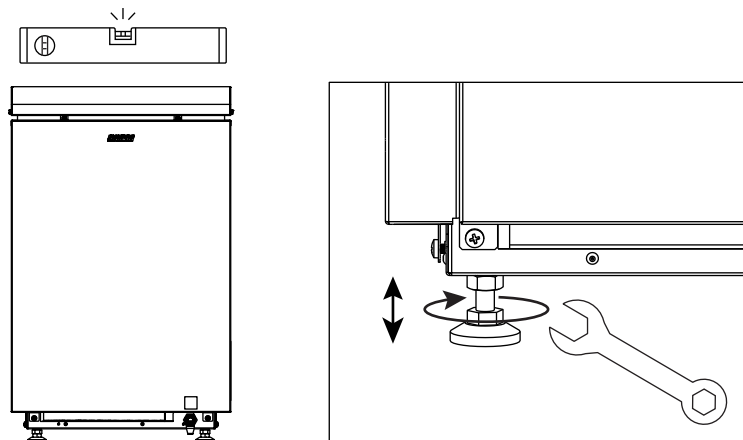
Рисунок 2. Установка каменки
