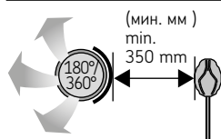
Рисунок 10. Минимальное расстояние от температурного датчика до вентиляционной отдушины.
