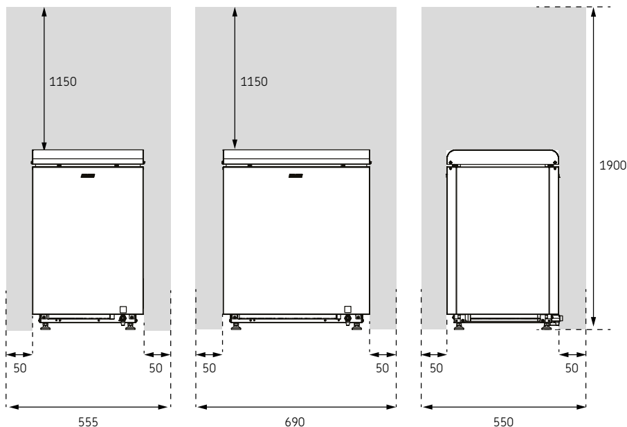
Kuva 1. Suojaetäisyydet
