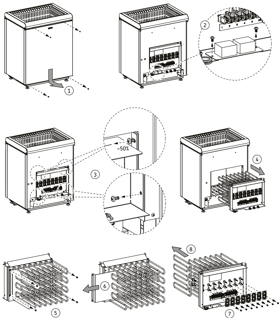
Figura 11. Sustitución de los elementos calefactores
