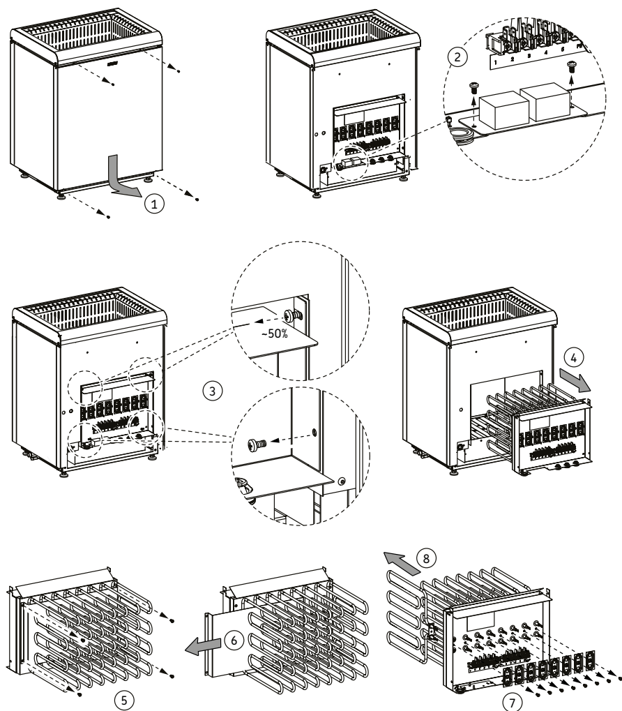
Figura 11. Sostituzione delle resistenze
