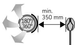
Figure 10. Distance minimale entre la bouche d'air et le capteur
