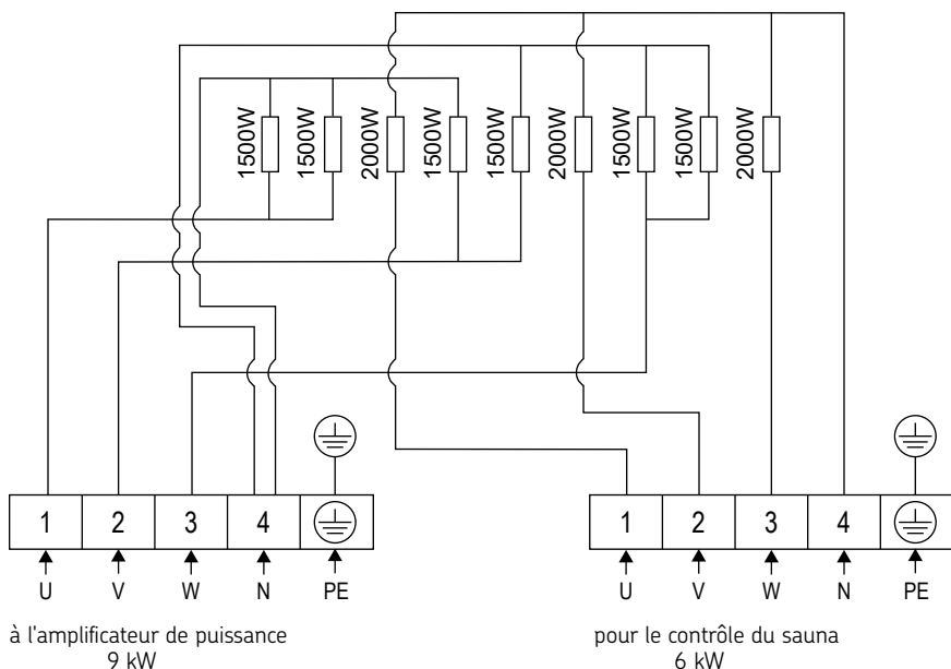
Figure 8. Schéma de câblage CR150E
