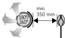
10 pav. Mažiausias atstumas nuo tiekiamo oro ventiliacijos angos iki temperatūros jutiklio
