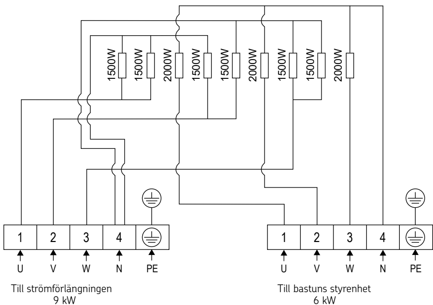
Bild 8. Kopplingsschema CR150E
