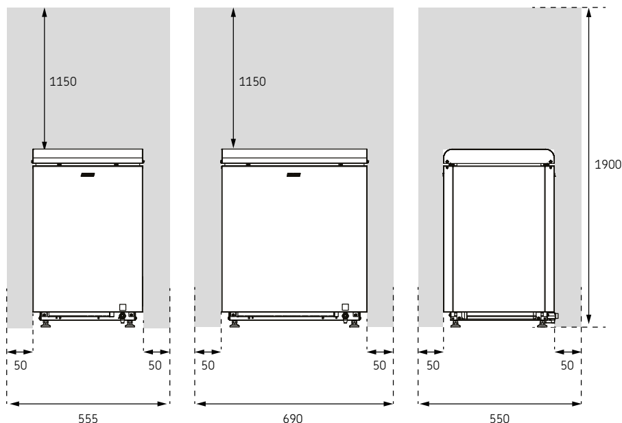
Figuur 1. Veiligheidsafstanden
