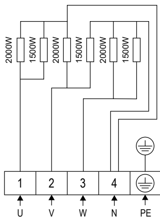
Bild 6. Kopplingsschema CR105E
