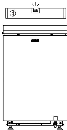
Kuva 2. Kiukaan asennus
