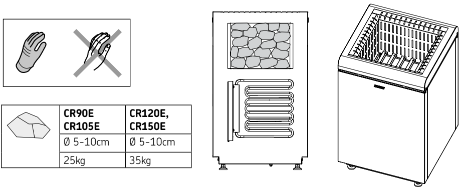
Figura 9. Colocación de las piedras de la sauna
