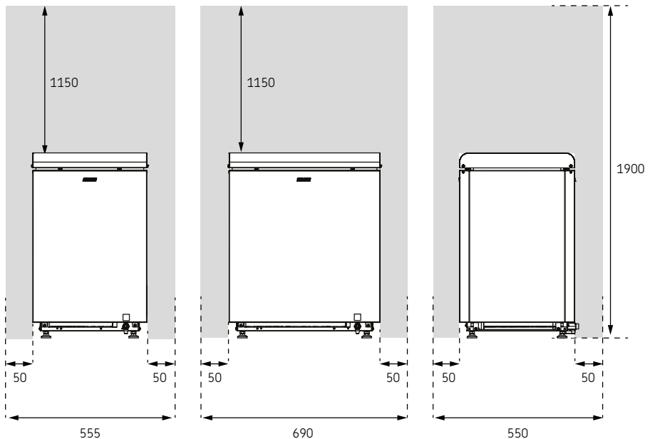
Abbildung 1. Sicherheitsabstände
