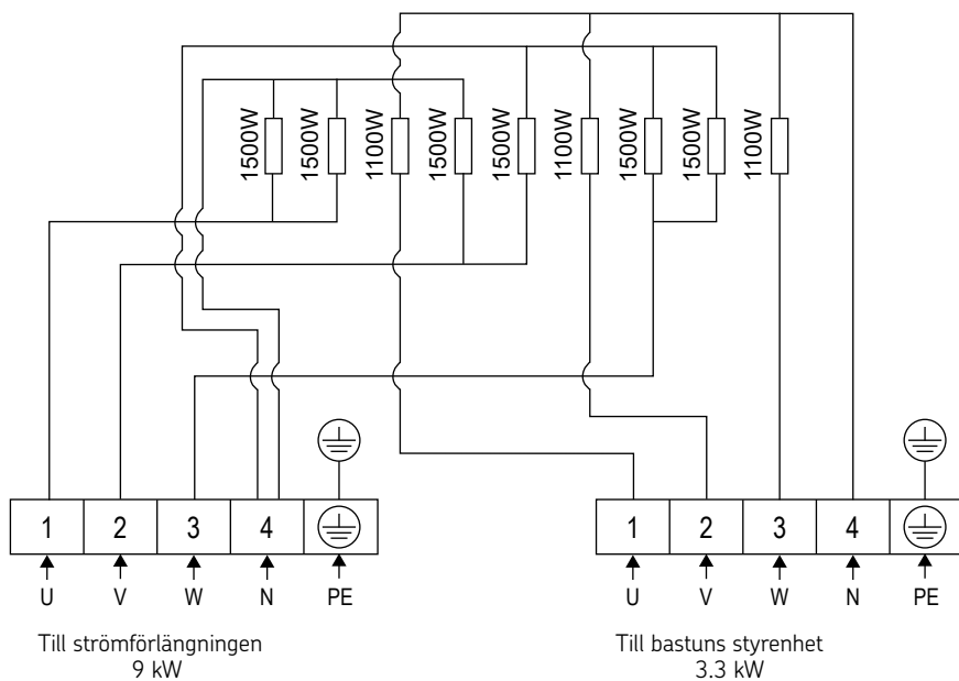
Bild 6. Kopplingsschema CR120E
