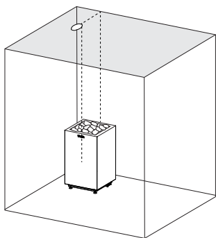
Bild 3b. Installera värmegivaren i taket
