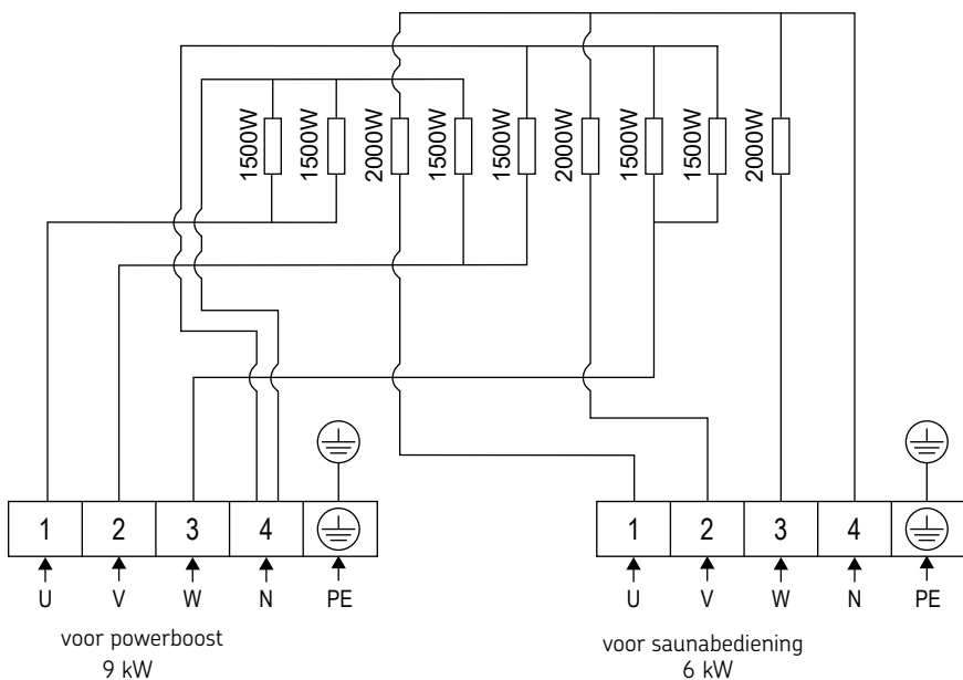
Figuur 8. Aansluitschema CR150E
