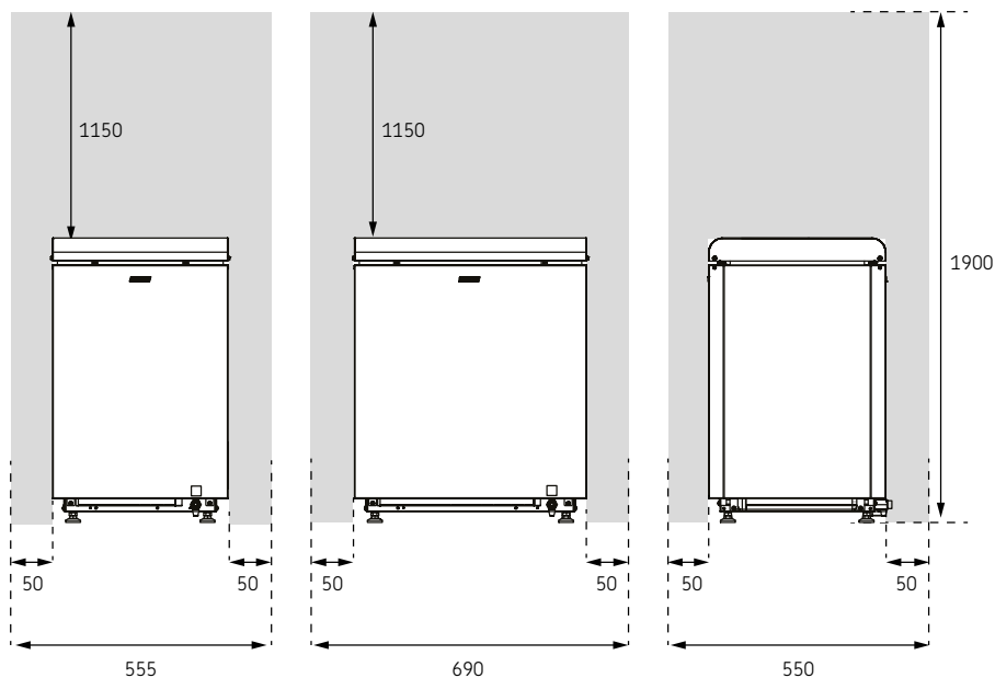
Joonis 1. Ohutuskaugused
