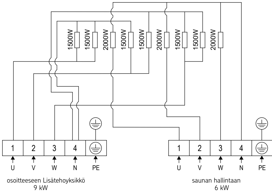
Kuva 8. Kytentäkaavio CR150E
