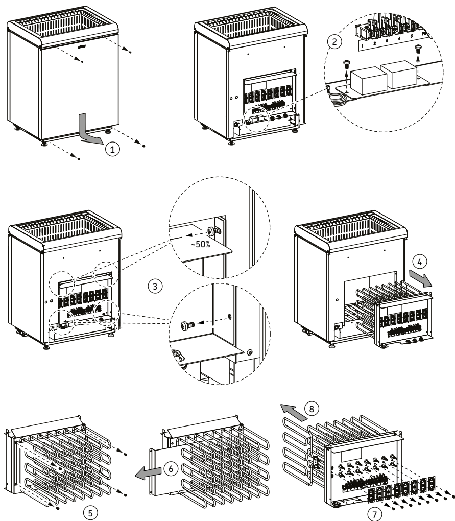
Bild 11. Byta värmeelement
