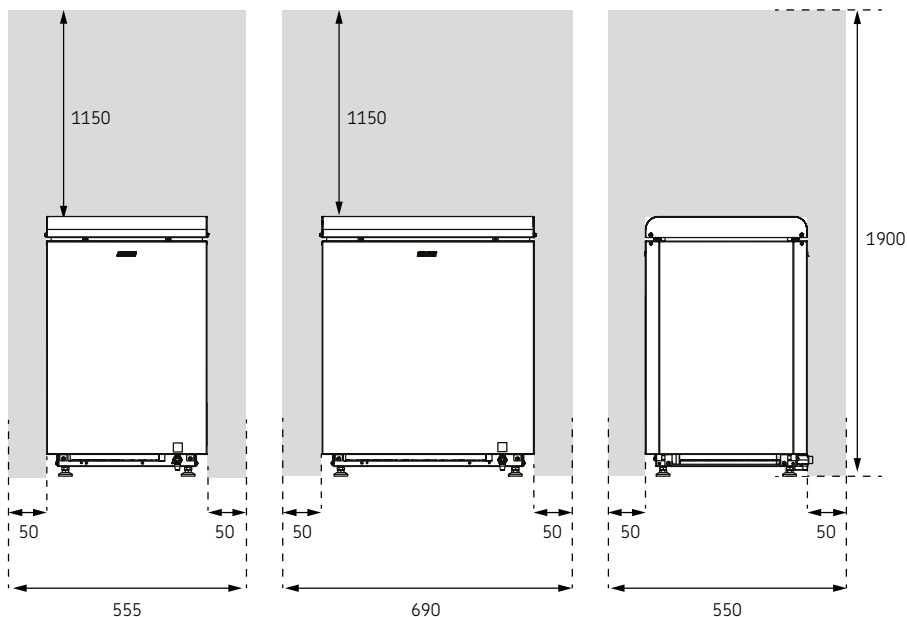
Bild 1. Säkerhetsavstånd
