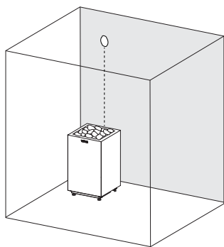
Bild 3a. Installera värmegivaren på väggen
