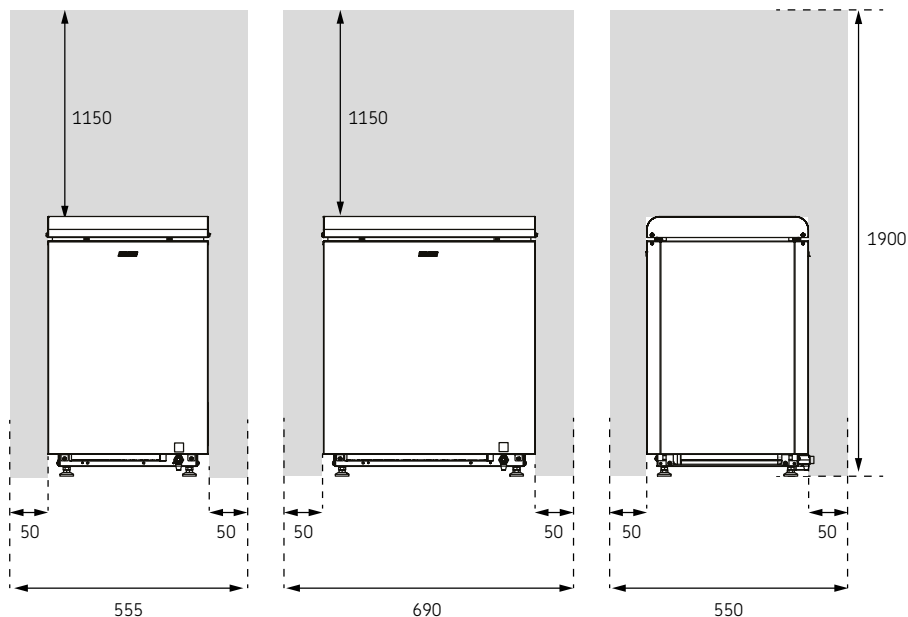
Slika 1. Varnostne razdalje
