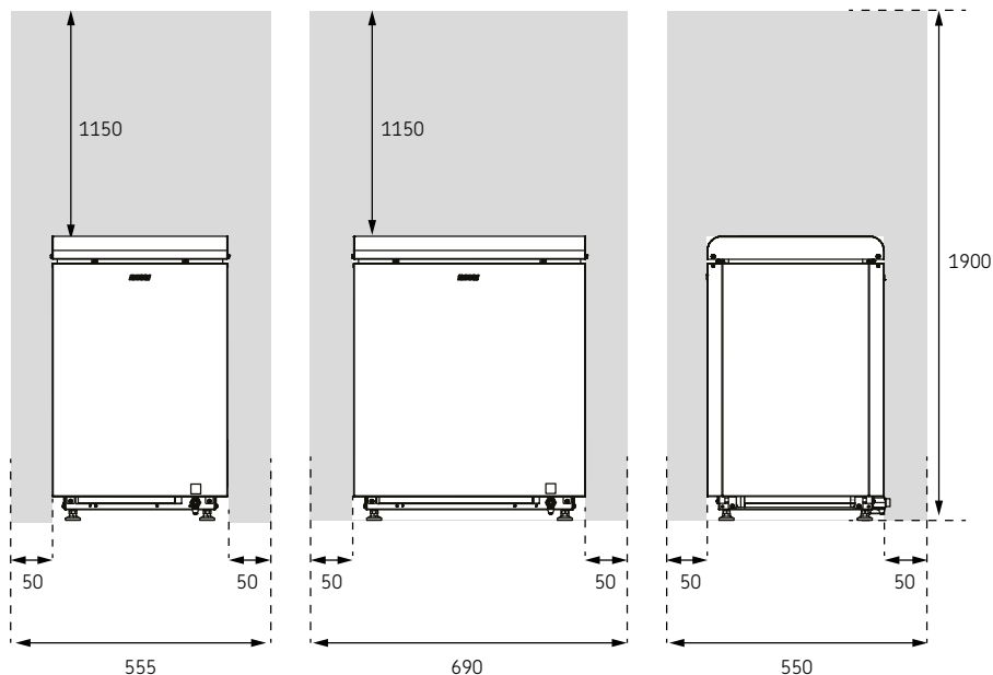
Obrázek 1 Bezpečnostní vzdálenosti
