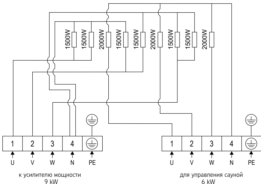
Рисунок 8. Электрическая схема CR150E
