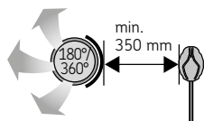
Figura 10. Distanza minima tra lo sfiato dell'aria di alimentazione e il sensore di temperatura.
