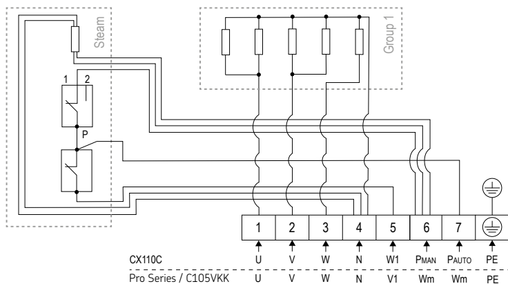
Bild 5. Kopplungsschema QU100S
