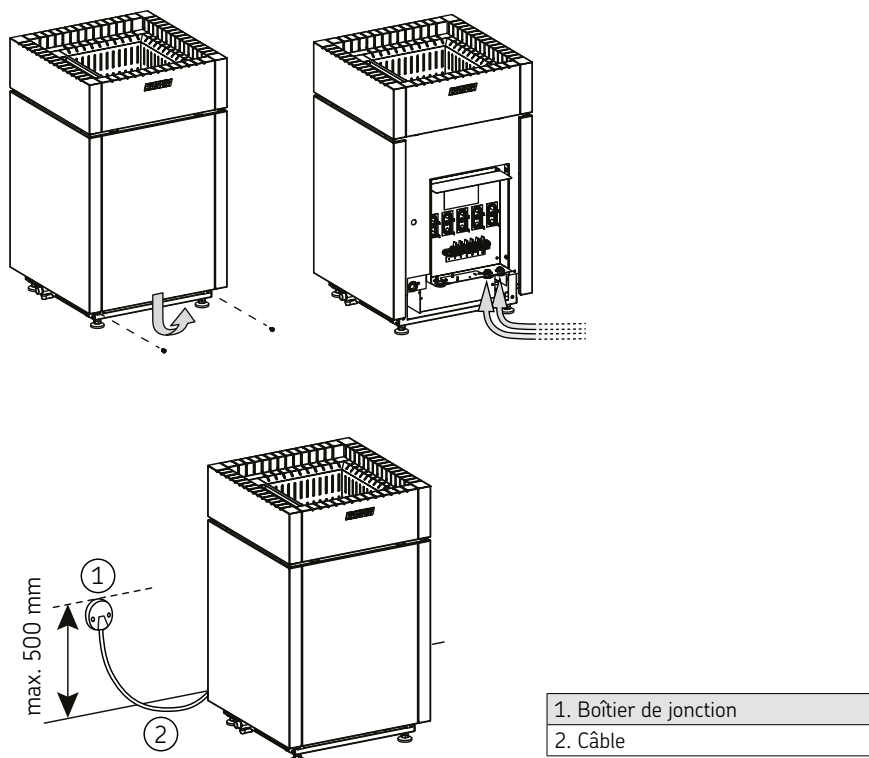
Figure 4. Raccordements électriques
