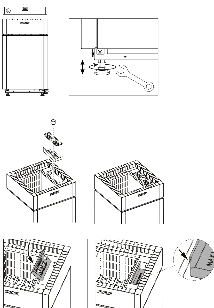
Kuva 2. Kiukaan asennus
