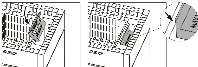
Рисунок 2. Установка каменки
